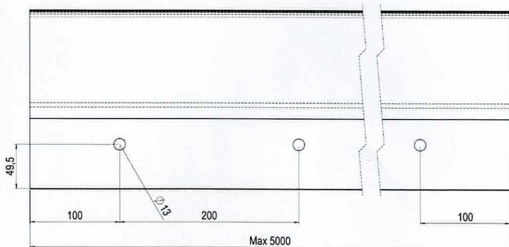
Abb. 4: Grundprofil ETP.002.11.AL.A Befestigung seitlich
