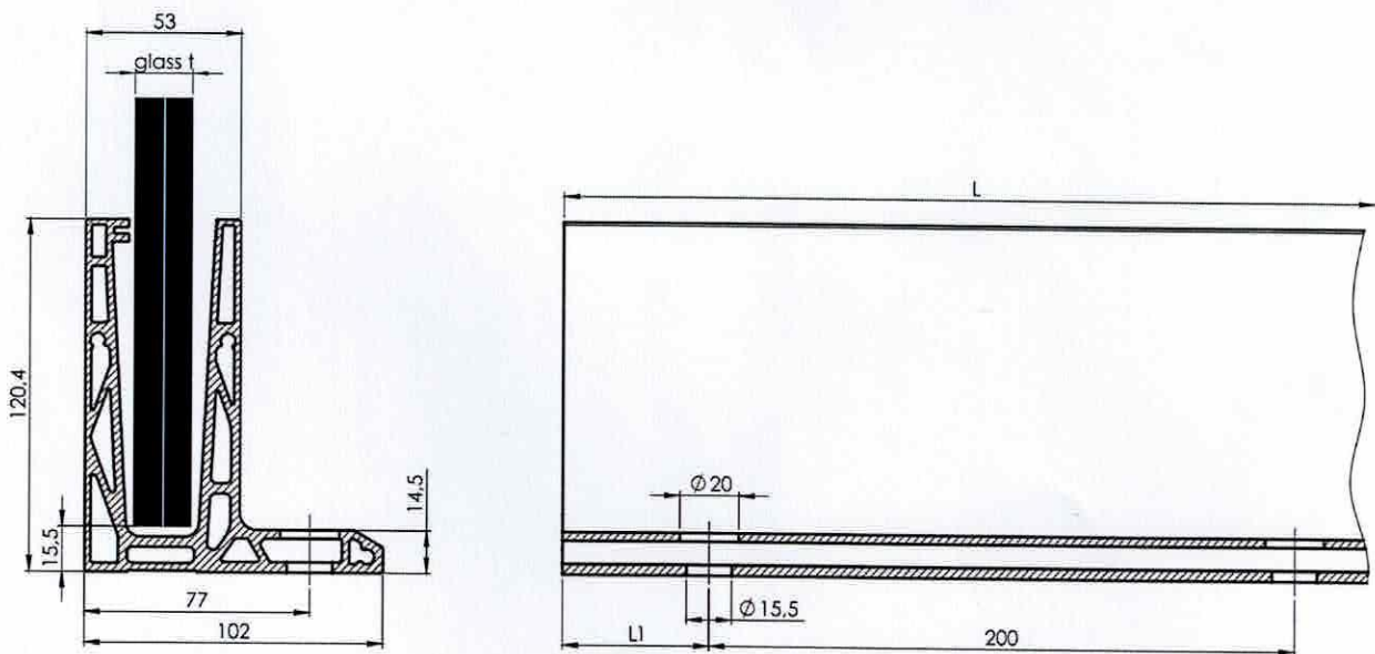
Abb. 6: Grundprofil ETP.006.03.AL.A Befestigung von oben
