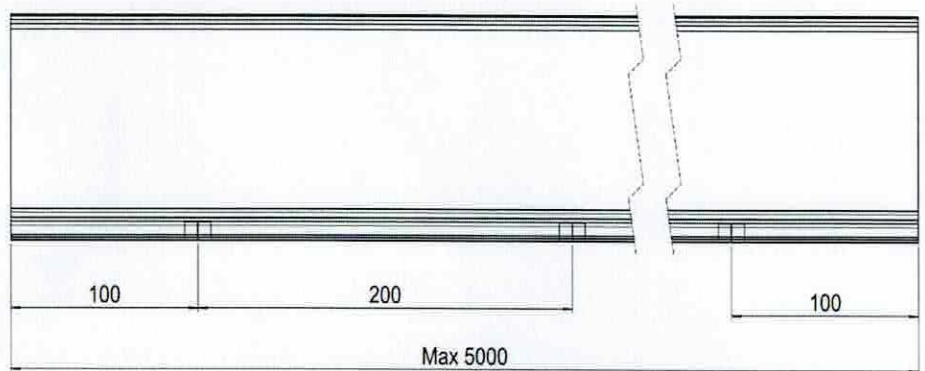
Abb. 3: Grundprofil ETP.002.03.AL.A Befestigung von oben
