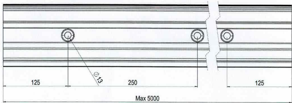
Abb. 2: Grundprofil ETP.002.02.AL.A Befestigung seitlich
