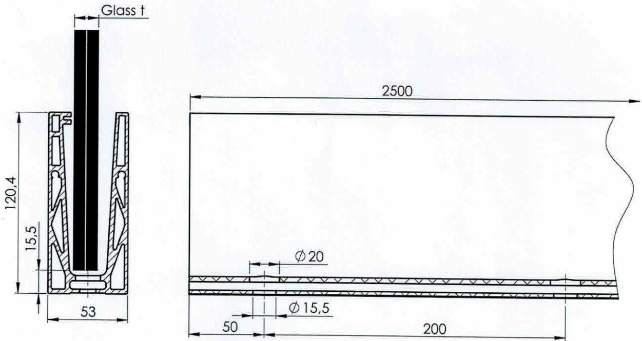
Abb. 5: Grundprofil ETP.006.01.AL.A Befestigung von oben
