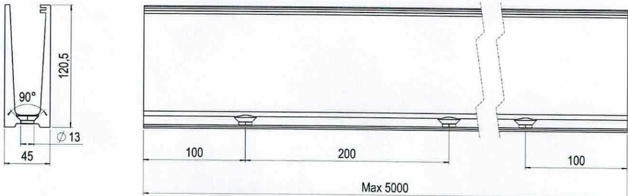
Abb. 1: Grundprofil ETP.001.01.AL.A Befestigung von oben
